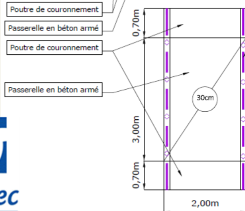
Vue en plan des passerelles au niveau des passages piétons
