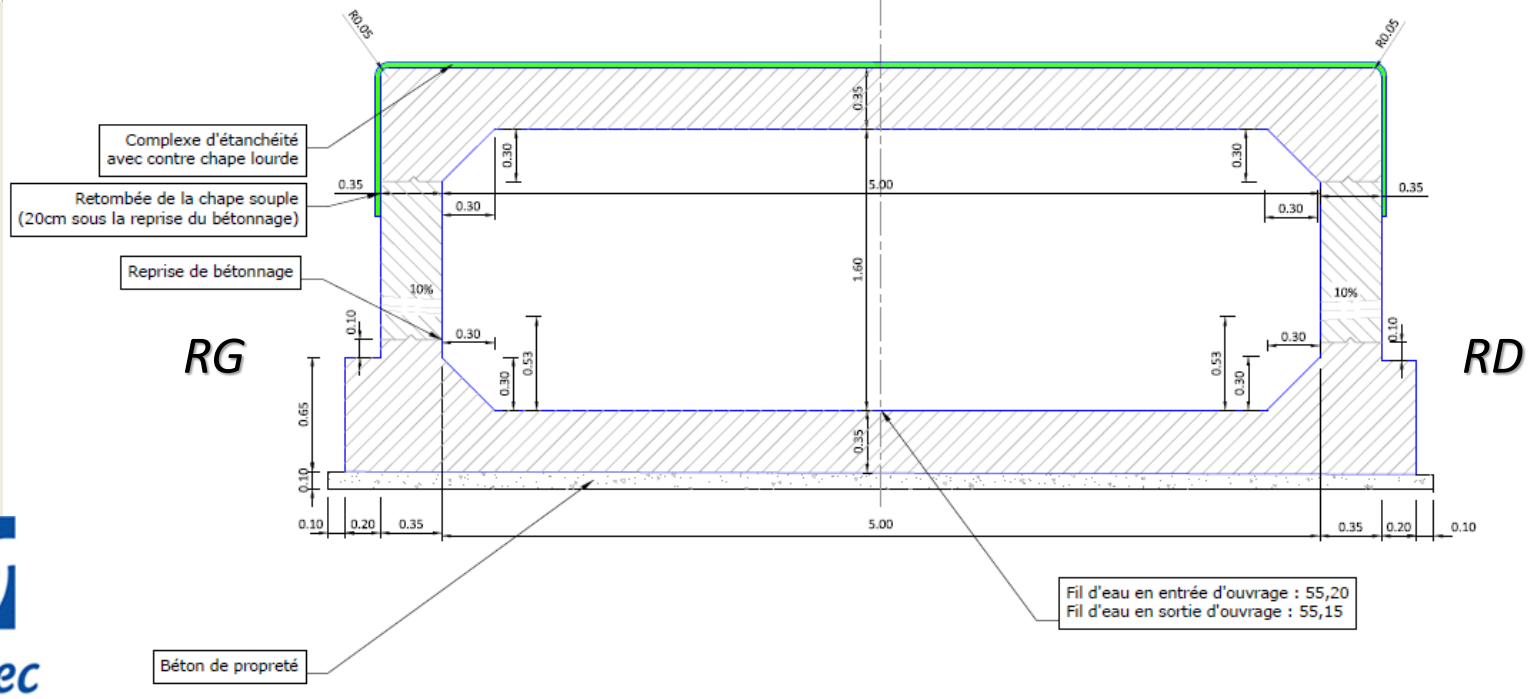
Ouvrage hydraulique au niveau de la Rue de la Reconnaissance
