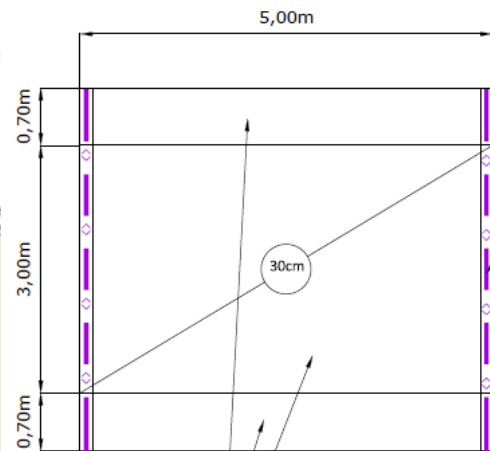
Vue en plan des passerelles au niveau des passages piétons
